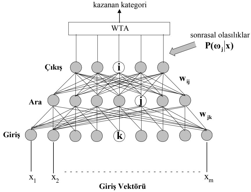
Şekil 4.5. Çok katmanlı ileri beslemeli sinir ağı sınıflandırıcısı [3].
