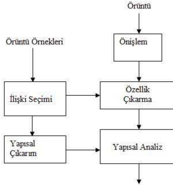
Şekil 2.3. Yapısal örüntü tanıma sistemi
