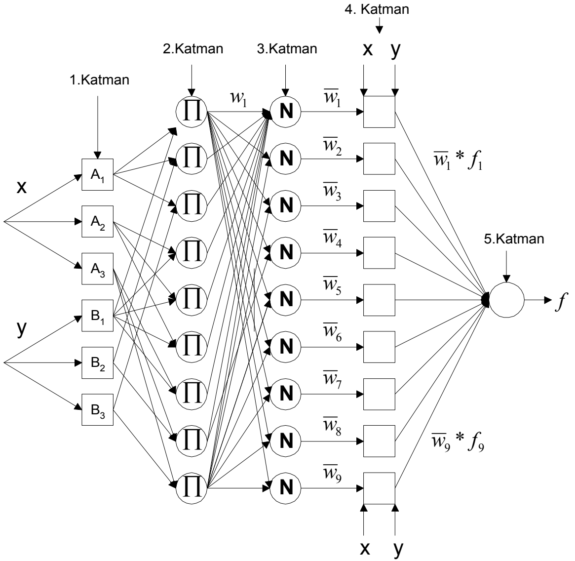
Şekil 4.6. 2 girişli 9 kurallı bir ANFIS sınıflandırıcı yapısı [2].
