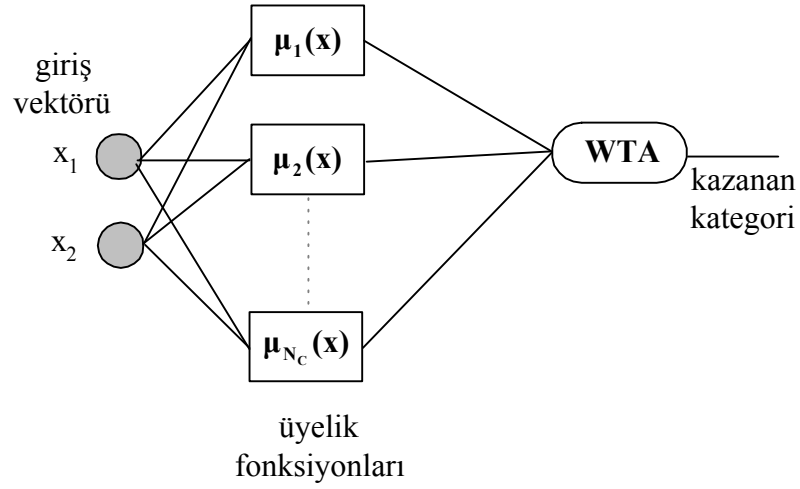
Şekil 4.2. Bulanık sınıflandırıcı [3].
