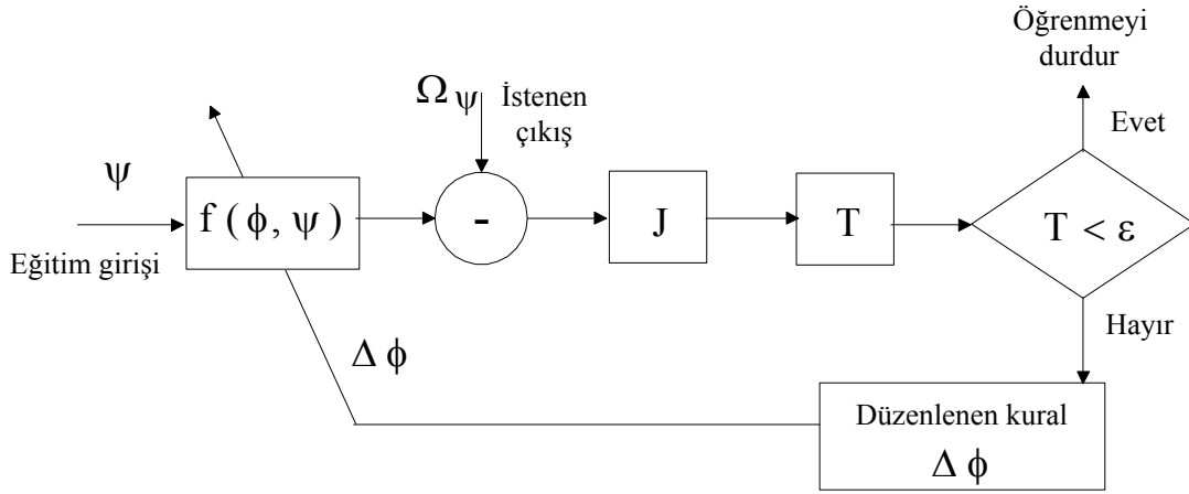
Şekil 2.5. Öğrenme süreci [3].
