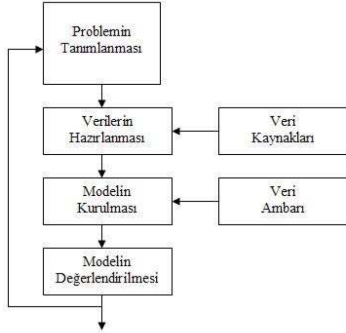
Şekil 3.3. Veri tabanlarında bilgi keşfi süreci ve veri madenciliği
