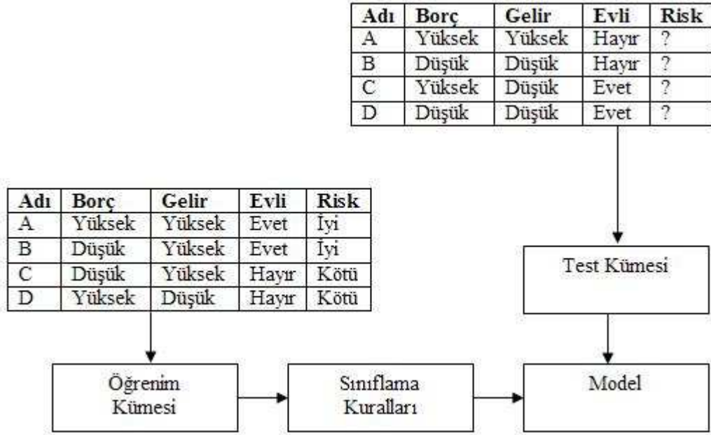
Şekil 3.4. Denetimli öğrenme
